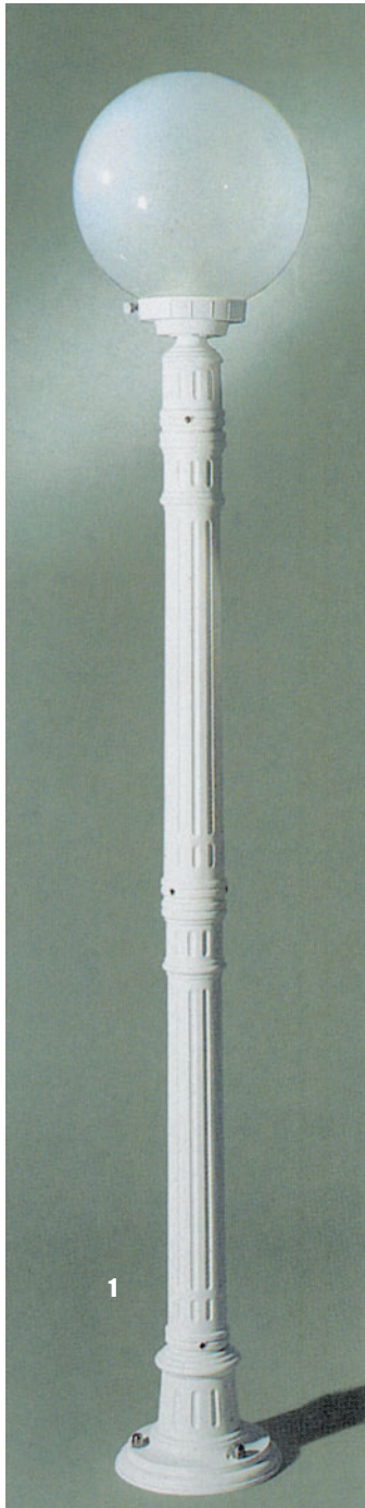
1 AL 11K/3153/B4 Weiß (Kopf) AL 11K/P012/B Weiß (Mast) H 152 cm Ø 25 cm 1xE27 max. 100W, IP23
