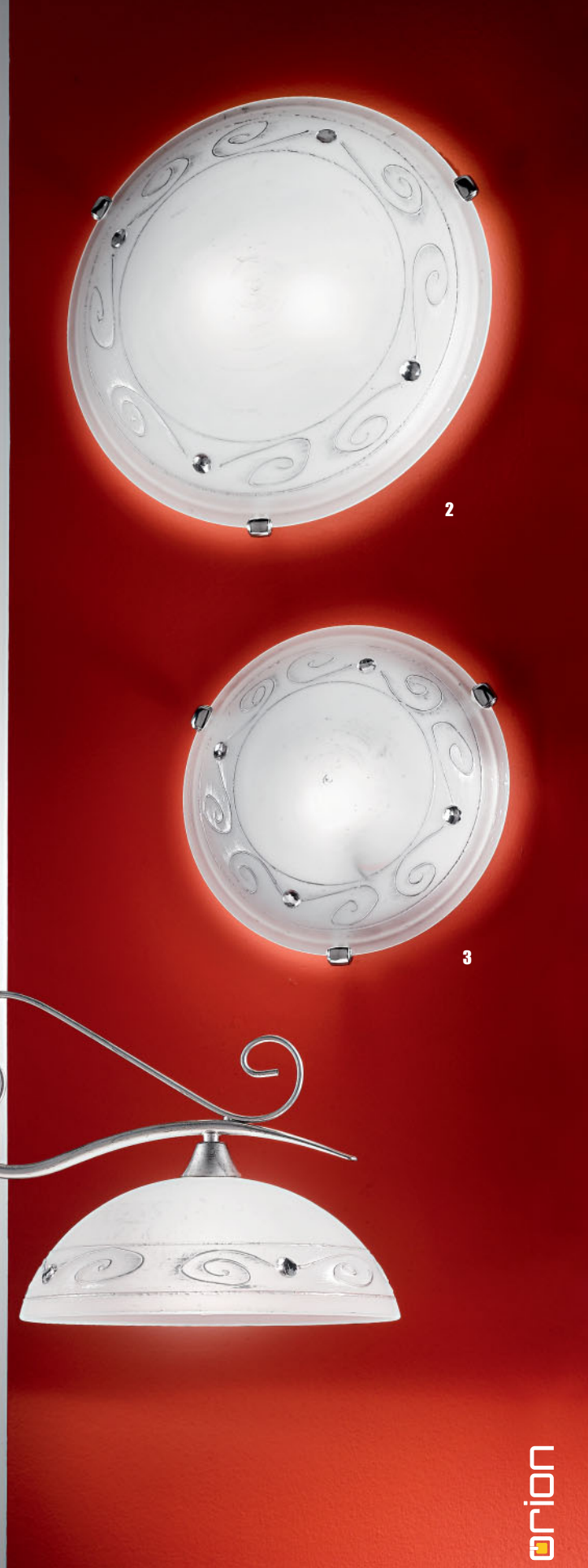
1 LU 1686/2 Antik-silber L 72 cm 2xE27 max. je 60W
