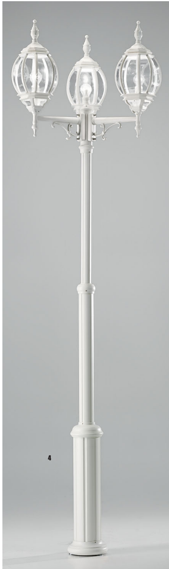
4 AL 11K/82899 Weiß H 265 cm Ø 65 cm 3xE27 max. je 100W IP43
